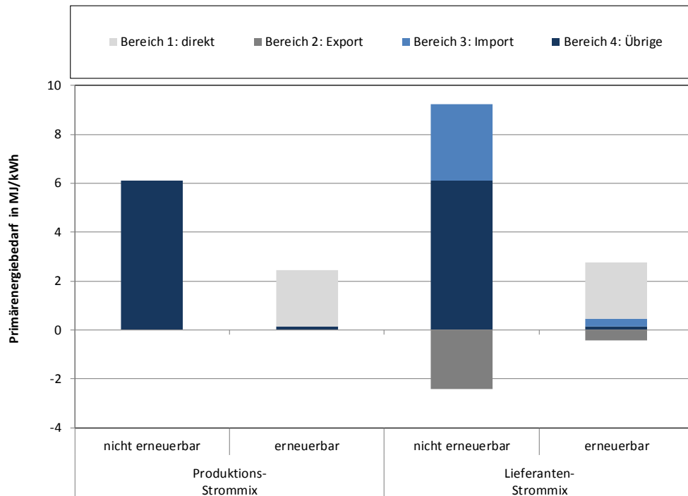
Fig. 6.2 Erneuerbarer und nicht erneuerbarer kumulierter Primärenergiebedarf des Schweizer Produktions- und Lieferanten-Strommixes in MJ pro kWh Strom aufgeteilt in die vier Bereiche. Die Zahlen und Anteile zum erneuerbaren und nicht erneuerbaren Primärenergiebedarf sind in Tab. I 2 und Tab. I 3 im Anhang aufgeführt.
